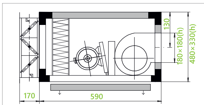
вентилятор с ременным приводом, клапаном и панельным фильтром Артикул для заказа А - 1213
