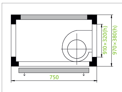
вентилятор с непосредственным приводом
