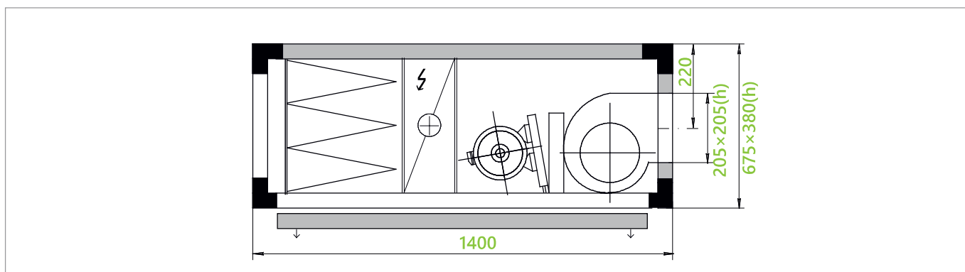
вентилятор с ременным приводом, карманным фильтром и электрическим нагревателем
