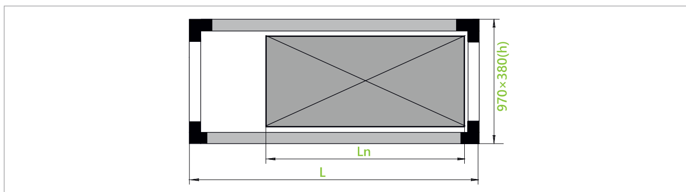
Блок шумоглушения с промежуточной секцией
