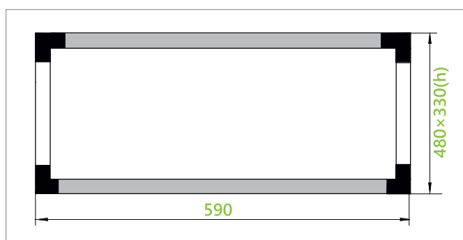
Промежуточная блок-секция
