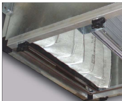
ПАНЕЛЬНЫЕ ФИЛЬТРЫ грубой очистки G3
