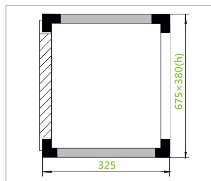
Блок-секция воздухораспределительная с решеткой
