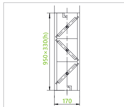
Клапан воздухозаборный утепленный GMK
