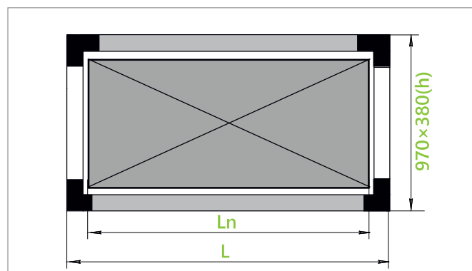
Блок шумоглушения без промежуточной секции
