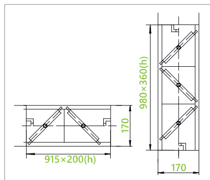
Клапан воздухозаборный REG
