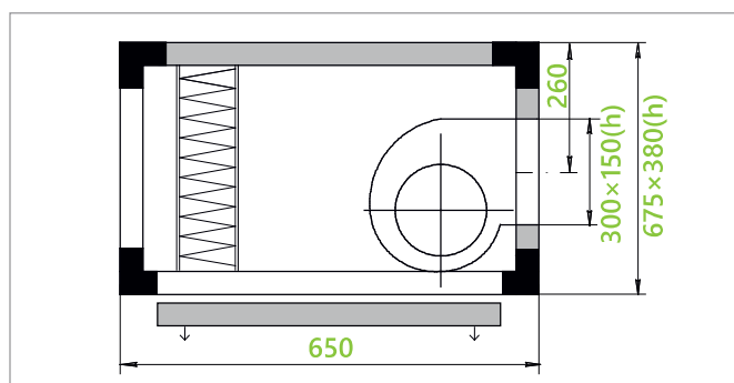
вентилятор с непосредственным приводом и панельным фильтром
