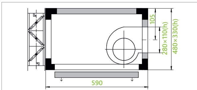
вентилятор с непосредственным приводом и клапаном
