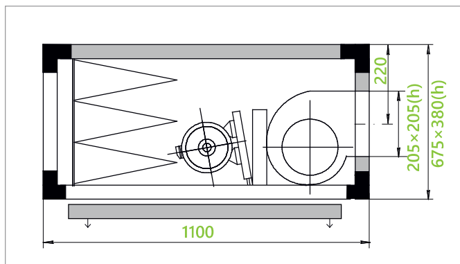
вентилятор с ременным приводом и карманным фильтром
