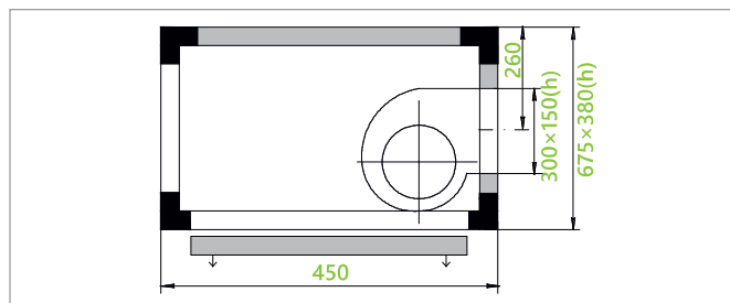
вентилятор с непосредственным приводом Артикул для заказа А - 2010
