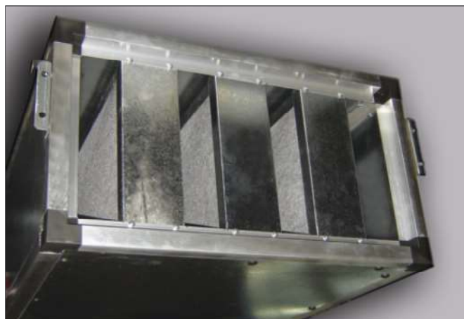
БЛОК ШУМОГЛУШЕНИЯ без промежуточной секцией
