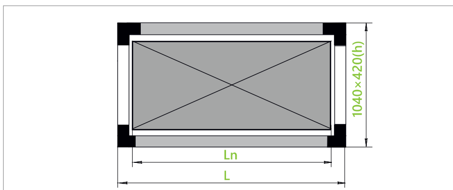
Блок шумоглушения без промежуточной секции
