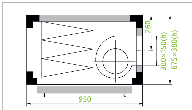
вентилятор с непосредственным приводом и карманным фильтром
