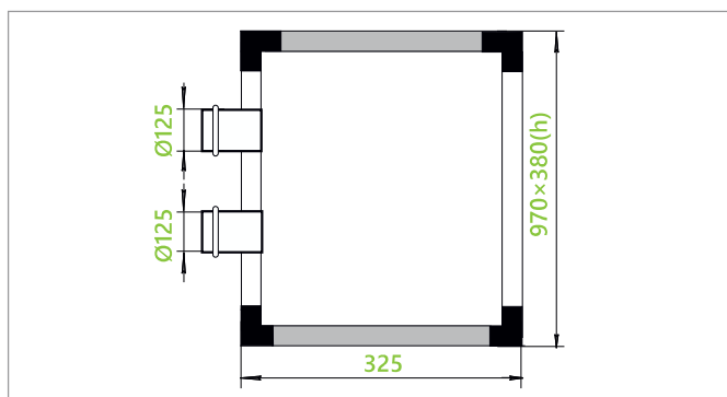
Блок-секция воздухораспределительная с 6-ю круглыми патрубками
