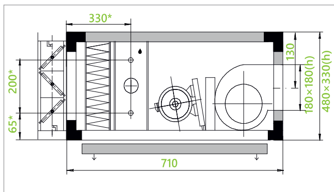
вентилятор с ременным приводом, клапаном, панельным фильтром и водяным нагревателем Артикул для заказа А - 1204 с двухрядным водяным нагревателем Артикул для заказа А - 1206 с трехрядным водяным нагревателем
