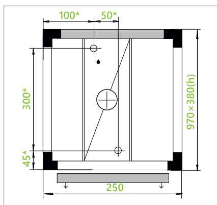
Блок воздухонагревателя водяного
