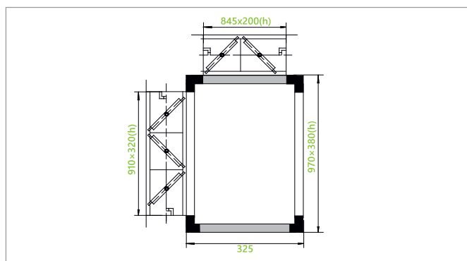
Блок-секция смесительная (сторона обслуживания "верх")
