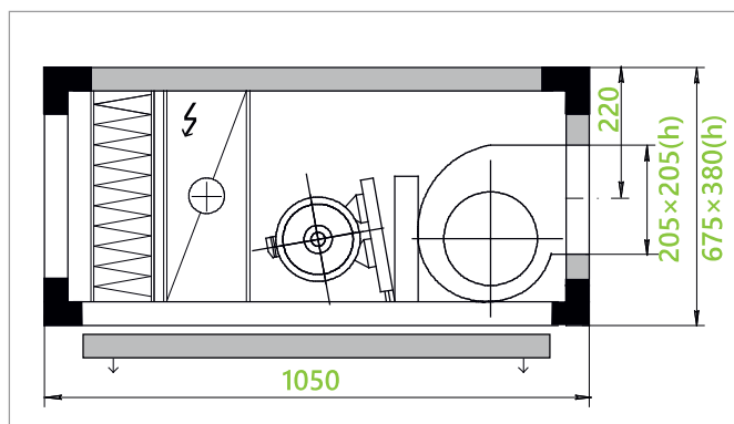
вентилятор с ременным приводом, панельным фильтром и электрическим нагревателем
