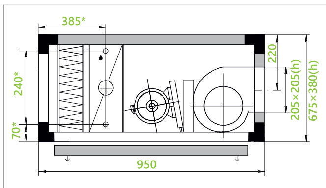
вентилятор с ременным приводом, панельным фильтром и водяным нагревателем
