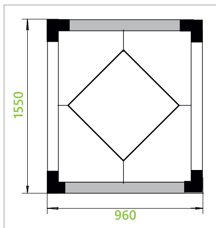
Блок пластинчатого теплоутилизатора
