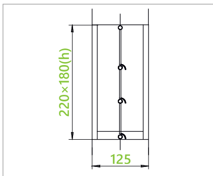
клапан обратный лепестковый KOL
