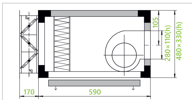
вентилятор с непосредственным приводом, клапаном и панельным фильтром Артикул для заказа А - 1214
