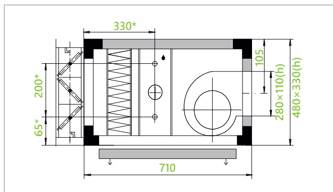
вентилятор с непосредственным приводом, клапаном, панельным фильтром и водяным нагревателем Артикул для заказа А - 1202 с двухрядным водяным нагревателем Артикул для заказа А - 1203 с трехрядным водяным нагревателем
