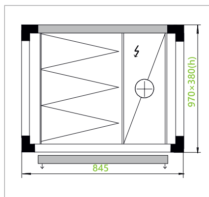
Блок очистки с электрическим нагревателем с карманным фильтром
