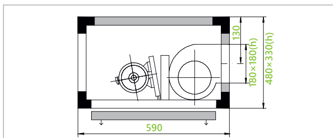
вентилятор с ременным приводом Артикул для заказа А - 1210
