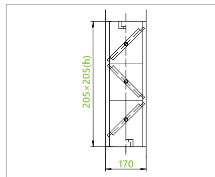
клапан воздухозаборный утепленный GMK
