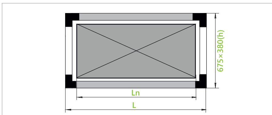
Промежуточная блок-секция
