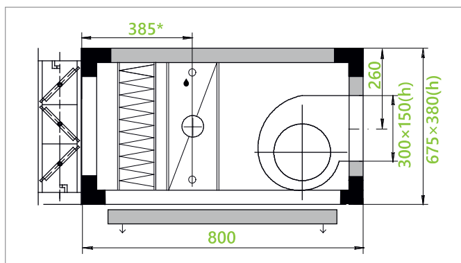
клапан и электропривод, вентилятор с непосредственным приводом, панельным фильтром и водяным трехрядным нагревателем Артикул для заказа А - 2031
