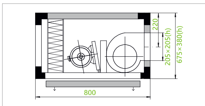
вентилятор с ременным приводом и панельным фильтром
