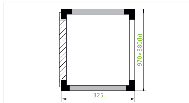
Блок-секция воздухораспределительная с решеткой
