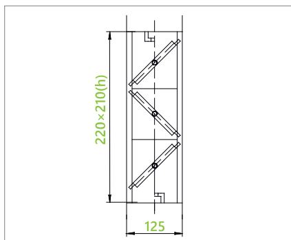
клапан воздухозаборный REL
