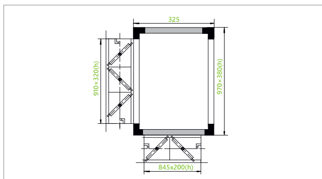
Блок-секция смесительная (сторона обслуживания "низ")
