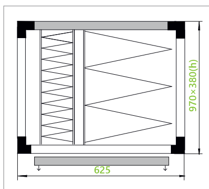
Блок фильтра карманного
