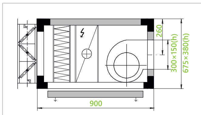
клапан и электропривод, вентилятор с непосредственным приводом, панельным фильтром и электрическим нагревателем 18 кВт Артикул для заказа А - 2041
