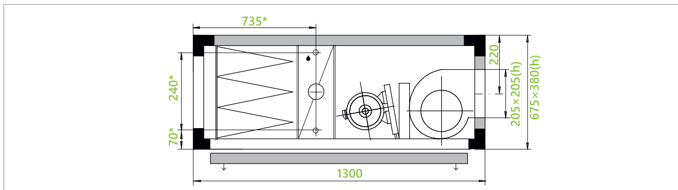
вентилятор с ременным приводом, карманным фильтром и водяным нагревателем
