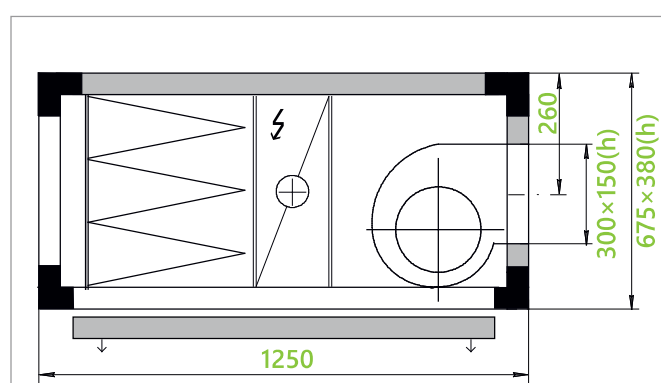
вентилятор с непосредственным приводом, карманным фильтром и электрическим нагревателем
