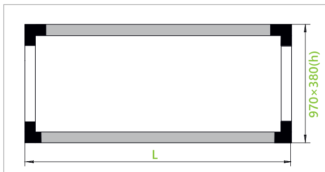
Блок-секция промежуточная
