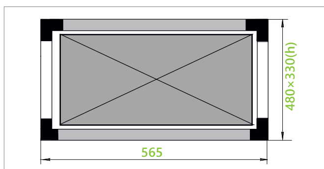
Блок шумоглушения без промежуточной секции
