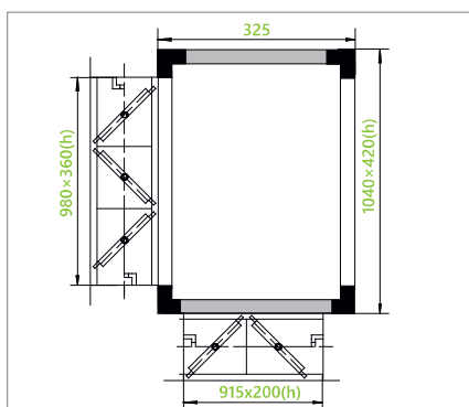
Блок-секция смесительная (сторона обслуживания "низ")
