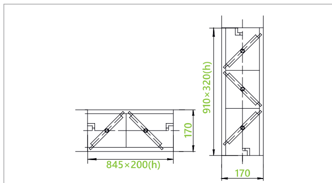
Клапан воздухозаборный REG горизонтальный и вертикальный
