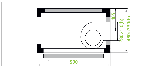
вентилятор с непосредственным приводом Артикул для заказа А - 1211
