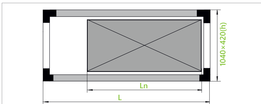
Блок шумоглушения с промежуточной секцией
