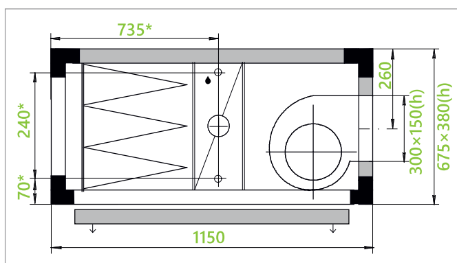
вентилятор с непосредственным приводом, карманным фильтром и водяным нагревателем
