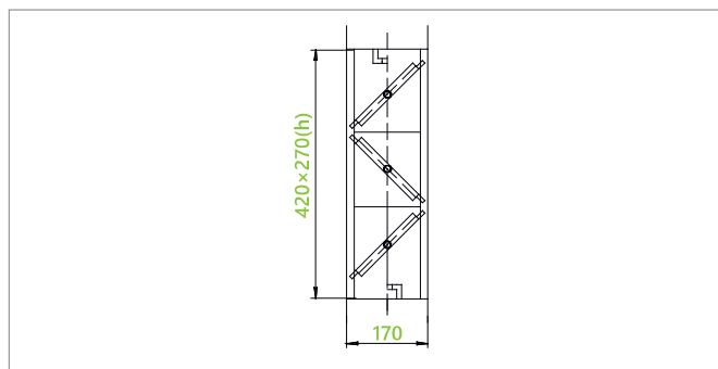
Клапан воздухозаборный REG
