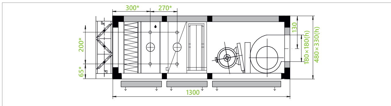
вентилятор с ременным приводом, клапаном, панельным фильтром, водяным нагревателем и фреоновым охладителем
