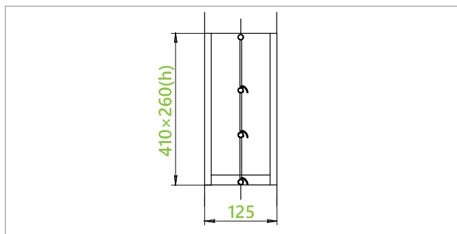
Клапан обратный лепестковый KOL
