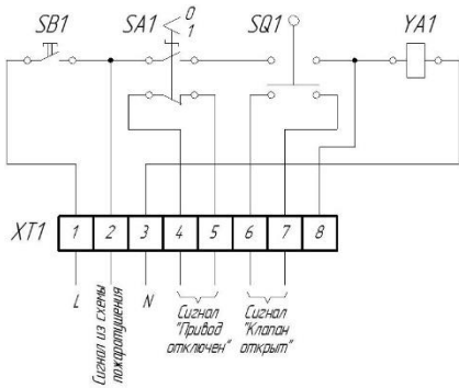
Рисунок 9 - Електрична схема електроприводу типу «відкрито/закрито»
