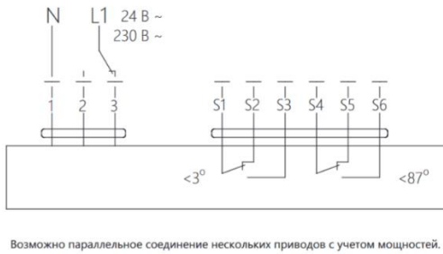
Рисунок 9 - Електрична схема електроприводу типу «відкрито/закрито»
