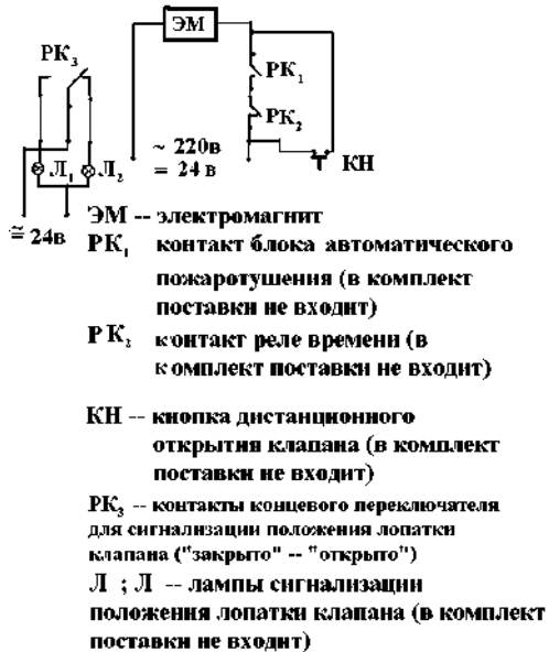
Рисунок 5 - Рекомендована схема включення клапанів KPU та сигналізації з електромагнітним приводом
