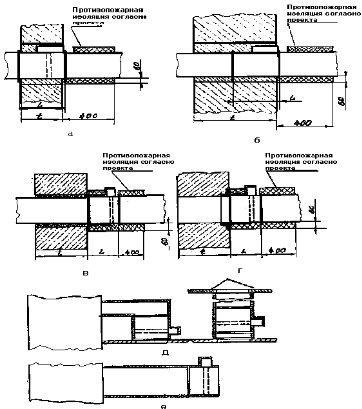
Рисунок 10 - Установчі схеми монтажу клапанів КРУ-1N
