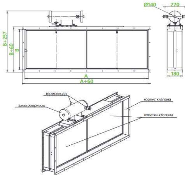
Рисунок 4 - Клапан KPU-1N вибухозахищений каналний прямокутний з електроприводом
