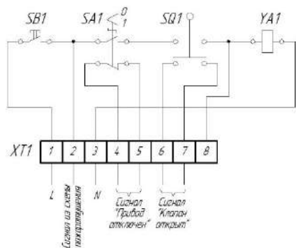
(для клапанів КРД, а також стінового димовидаляючого виконання КРУ) Рисунок 9 - Електрична схема включення клапанів та сигналізації з електромагнітним приводом
