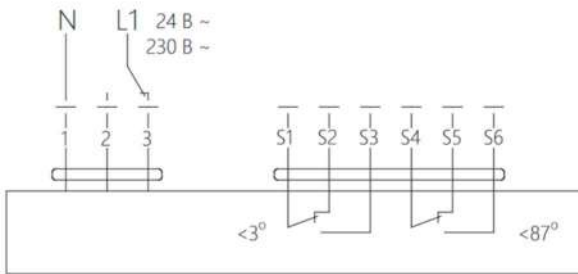
Рисунок 7 - Електричні схеми підключення клапана KPU з електроприводом
