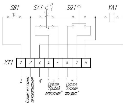
Рисунок 7 - Схема електричних з'єднань виконавчого механізму з електромагнітом Діаграма роботи контактів
