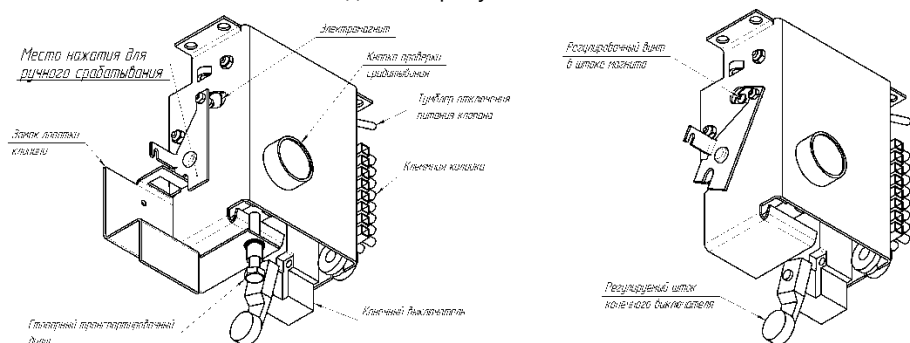
Рисунок 5 - Места регулирования исполнительного механизма с магнитом
