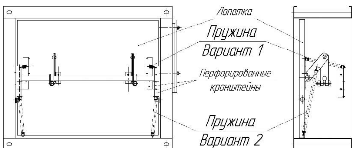
Рисунок 6 - Варианты встановлення пружин
