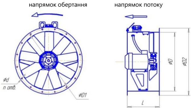
Рисунок 1 Загальний вид вентилятора типу OZA-201
