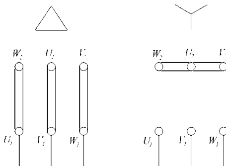
Рисунок 2 – Схема підключення електродвигуна до мережі живлення 380 В
