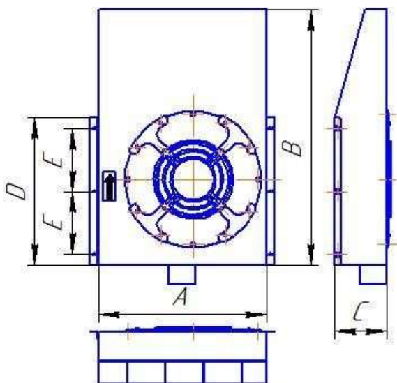
Рисунок 1 Загальний вид вентилятора типу типу RJF-DU
