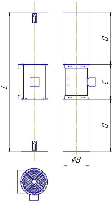
Рисунок 2 Загальний вид вентилятора типу типу JF-DU
