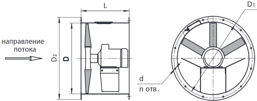
Рисунок 1 – Габаритные, присоединительные и установочные размеры вентилятора OZA-DUV
