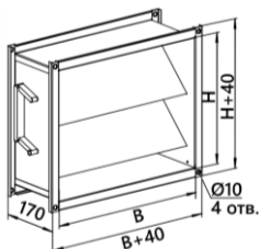
Рисунок 1 - Загальний вид клапана типу KP-REG
