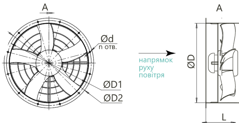
Рисунок 1 - Рисунок 1 Загальний вид вентилятора типу C-OZA-C
