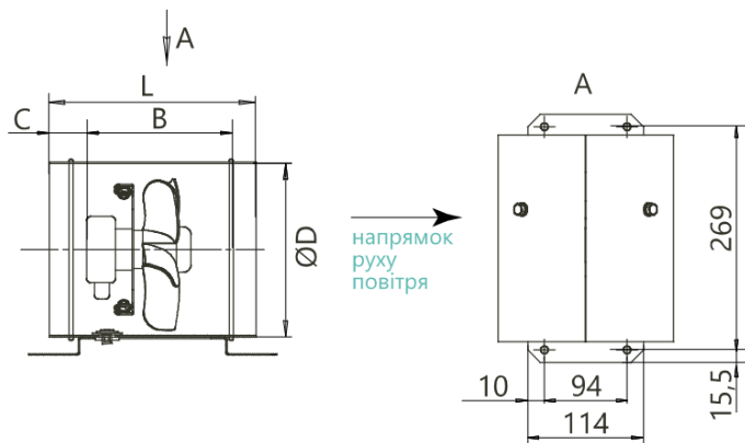
Рисунок 1 - Рисунок 1 Загальний вид вентилятора типу C-OZA-T
