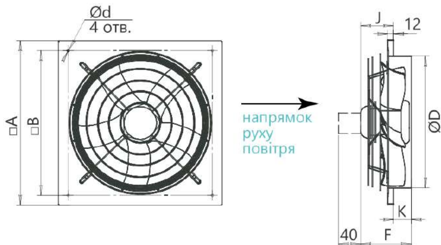
Рисунок 1 - Рисунок 1 Загальний вид вентилятора типу С-ОЗА-Р
