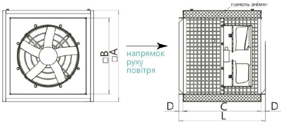
Рисунок 1 - Рисунок 1 Загальний вид вентилятора типу C-OZA-S
