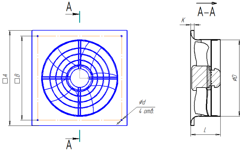
Рисунок 1. Габаритные, присоединительные и установочные размеры вентиляторов С-ОЗА-Р(Канал-ОСА-П)
