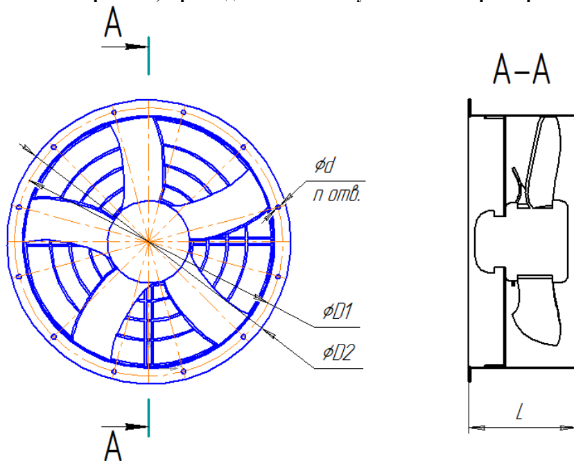
Рисунок 1. Габаритные, присоединительные и установочные размеры вентиляторов С-OZA-C
