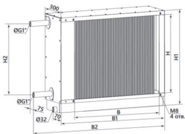
Рисунок 1 - Загальний вид повітроохолоджувача типу С-VKO
