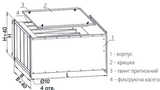
Рисунок 1 - Загальний вид фільтра типу C-FKP
