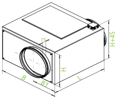
Рисунок 1 - Рисунок 1 Загальний вид вентилятора типу C-VENT-PB-S
