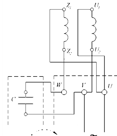
Рисунок 3 - Схема підключення вентилятора до ланцюга живлення 220 В
