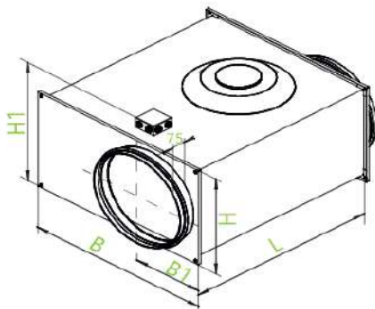
Рисунок 1 - Рисунок 1 Загальний вид вентилятора типу C-VENT-PF-EX
