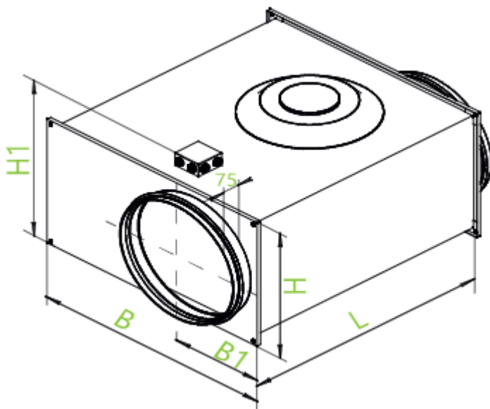
Рис. 1 Основные размеры вентиляторов С-VENT-PF-EX
