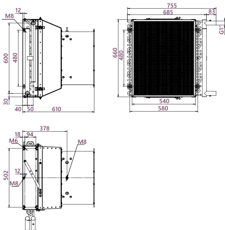
Рисунок 2 - Габаритні та приєднувальні розміри AVN-A
