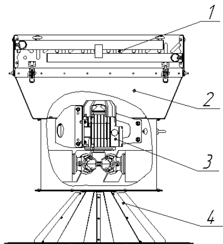
1 – теплообмінник; 2 – захисний кожух; 3 – вентилятор; 4 – повітророзподільник Рисунок 1 - Загальний вид агрегату типу AVN-A
