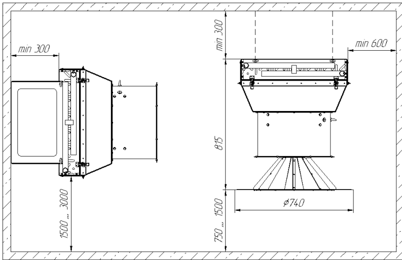
Рисунок 3 - Рекомендовані схеми встановлення AVN-A
