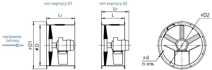
Рисунок 1 Загальний вид вентилятора типу OZA-301
