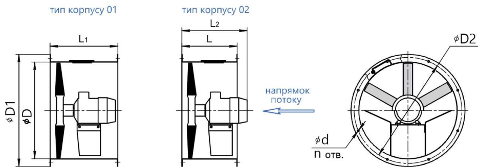
Рисунок 1 Загальний вид вентилятора типу OZA-HD
