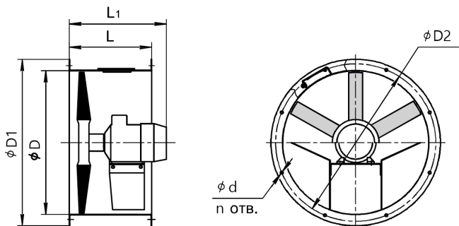
Рисунок 1 Загальний вид вентилятора типу OZA-RV
