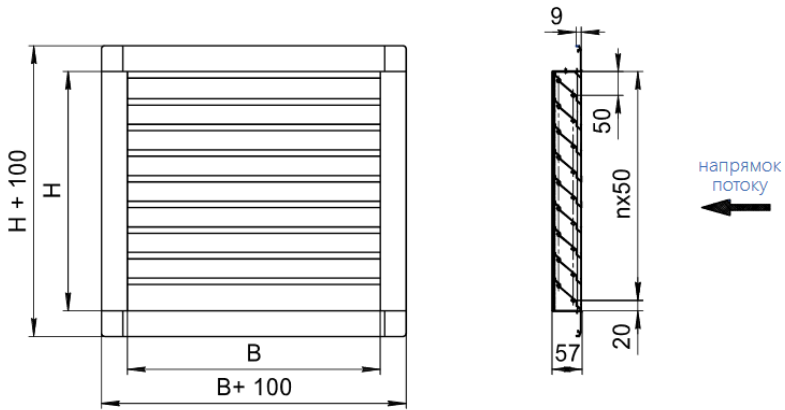
Рисунок 1 Загальний вид решітки типу OZA-R50
