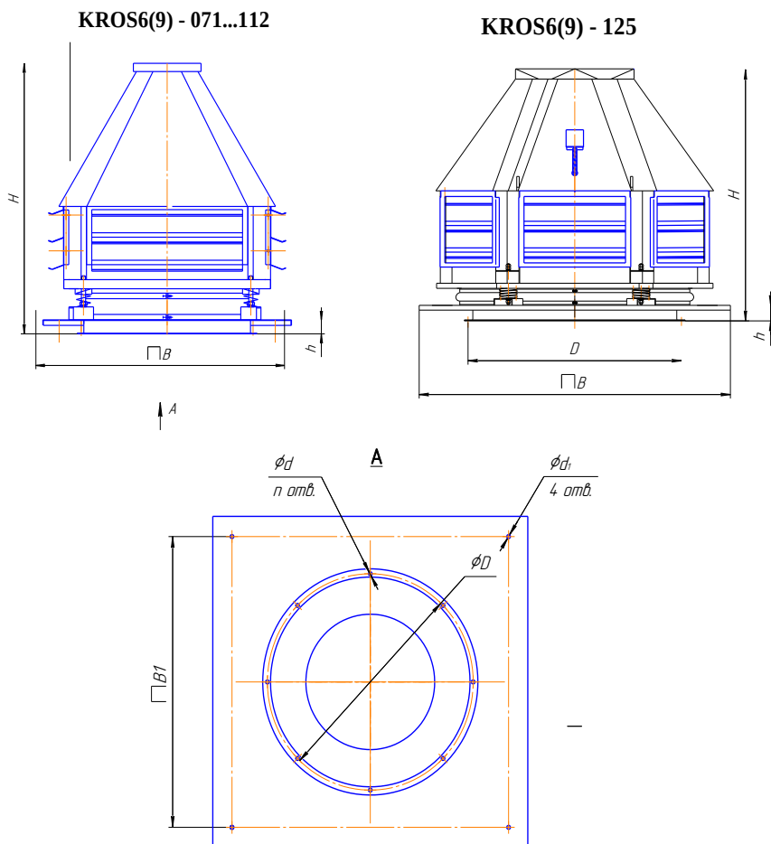
Рисунок 2. Вентилятор даховий KROS6 (9) – 071...125
