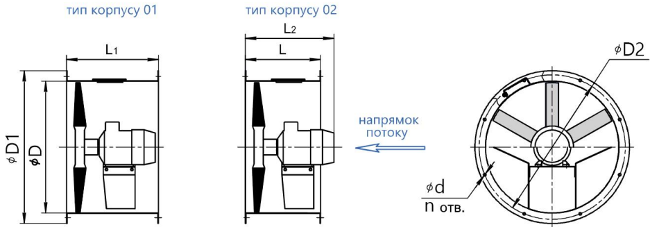
Рисунок 1 Загальний вид вентилятора типу OZA-HD
