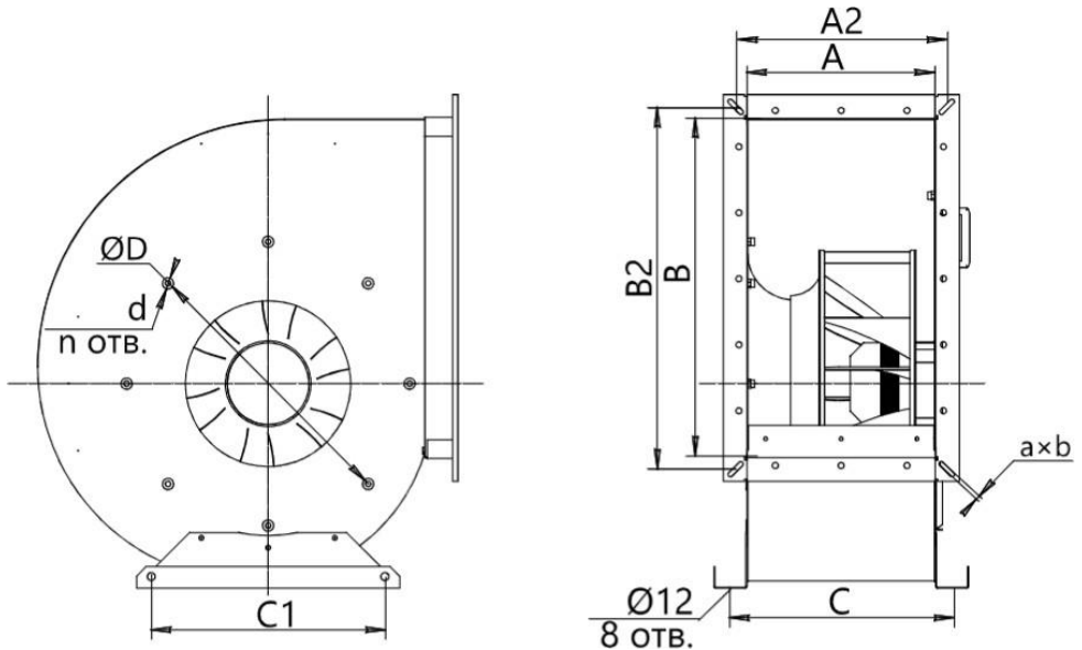
Рис.1 – Габаритные и присоединительные размеры RAV
