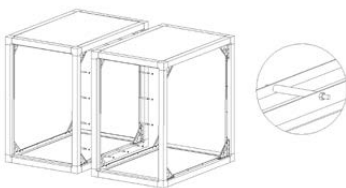
Болтове з'єднання каркаса
