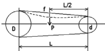
Рисунок 6. Контроль натяжіння.
