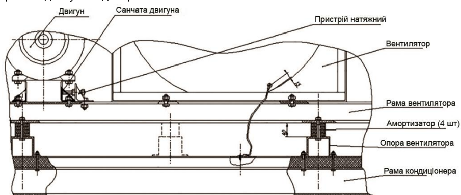
Рисунок 5. Регулювання натяжіння ременів вентилятора блока
