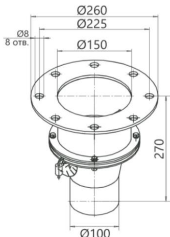
Рисунок 1 - Клапан витратомір-відсікач К-РВ
