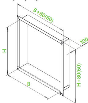
Рисунок 1 Загальний вид рами типу SET
