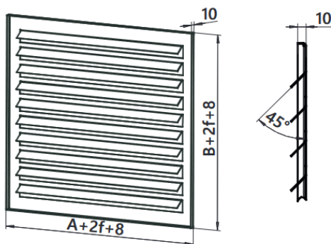
Рисунок 1 Загальний вид решіток типу RES
