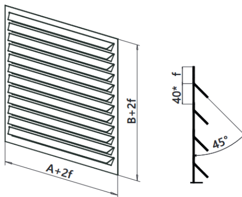
Рисунок 1 Загальний вид решіток типу RES
