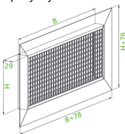
Рисунок 1 Загальний вид решіток типу RKP
