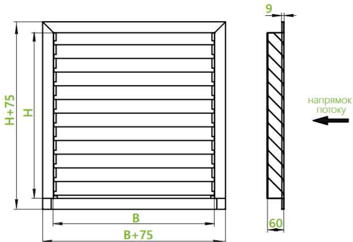
Рисунок 2 Загальний вид решітки типу RO50
