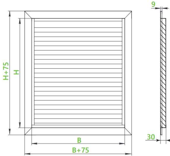
Рисунок 1 Загальний вид решітки типу RO25
