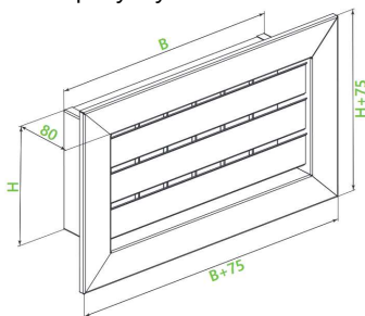
Рисунок 1 Загальний вид решіток типу RRD-25
