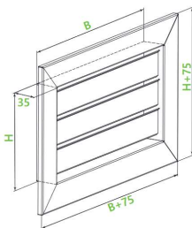
Рисунок 1 Загальний вид решітки типу RRO-25
