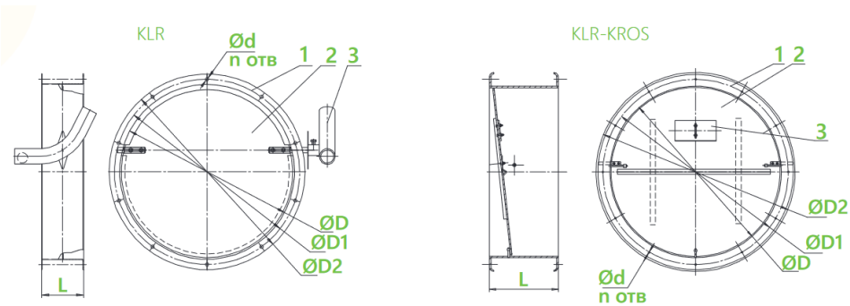
Рисунок 2 Загальний вид клапанів типу KLR круглого перерізу
